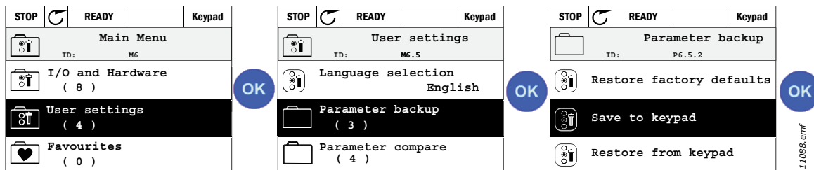
Рис. 6. Копирование параметров
