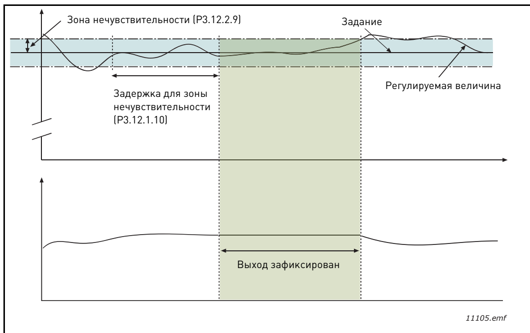
Рис. 33. Зона нечувствительности
